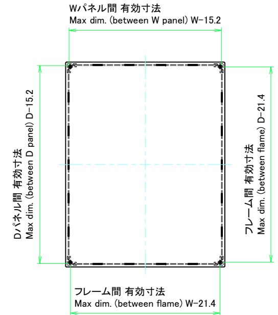
下カバー / Bottom cover
