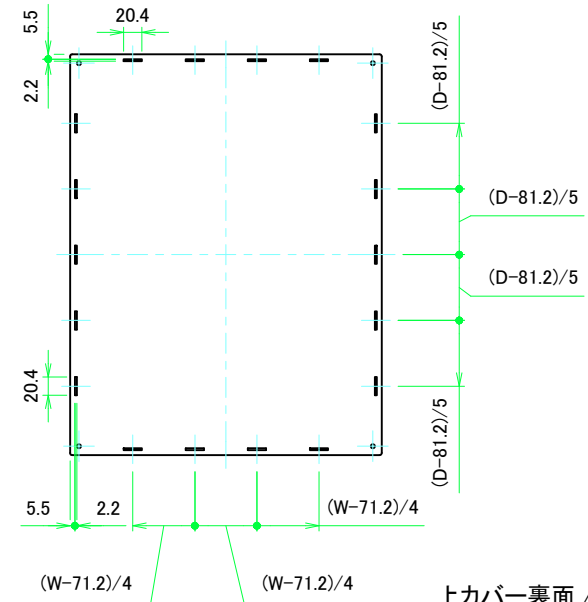
上カバー裏面 / Top cover Backside
